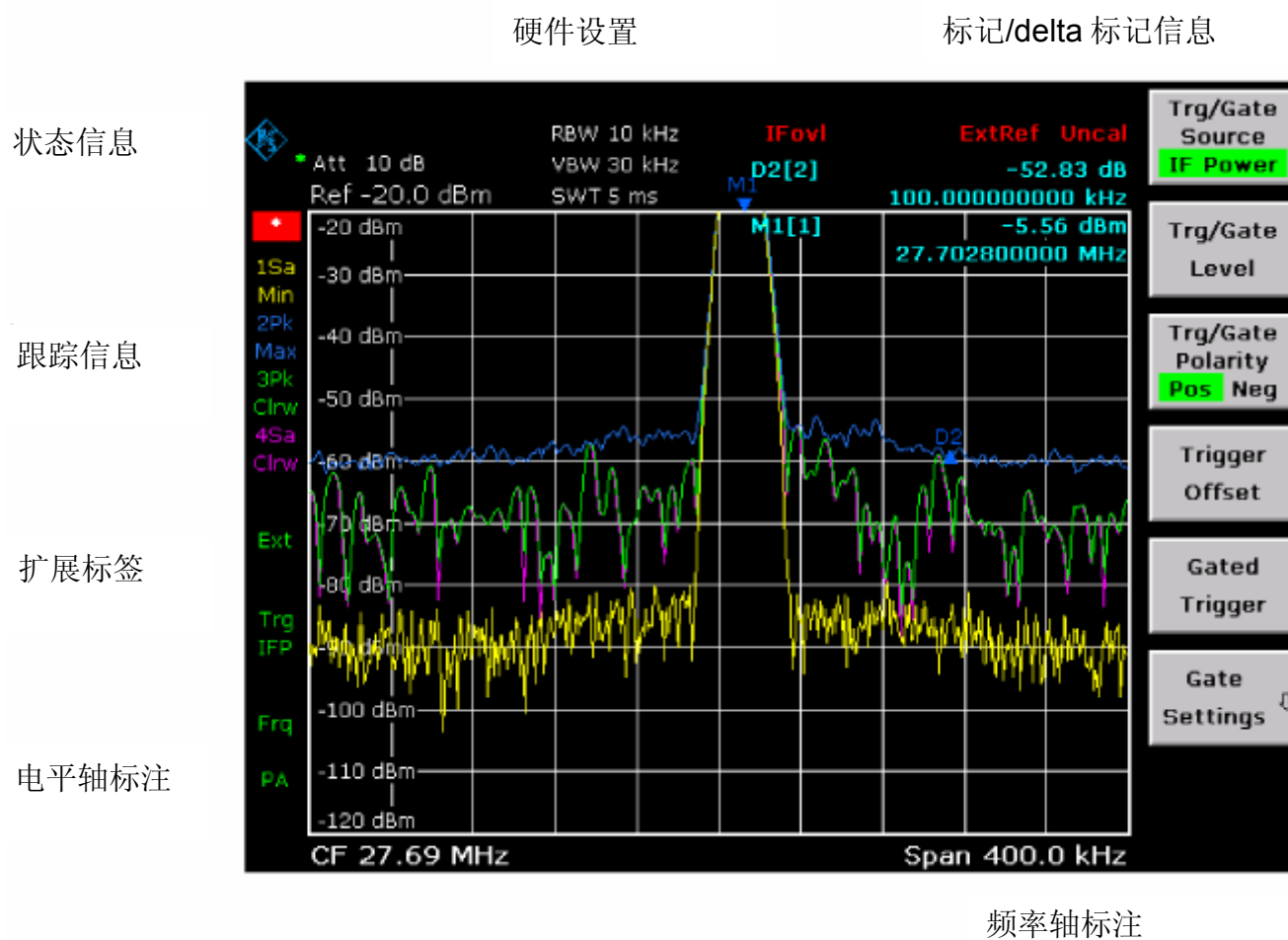
图 4-1 分析仪操作过程中R&S FSL的屏幕布局
