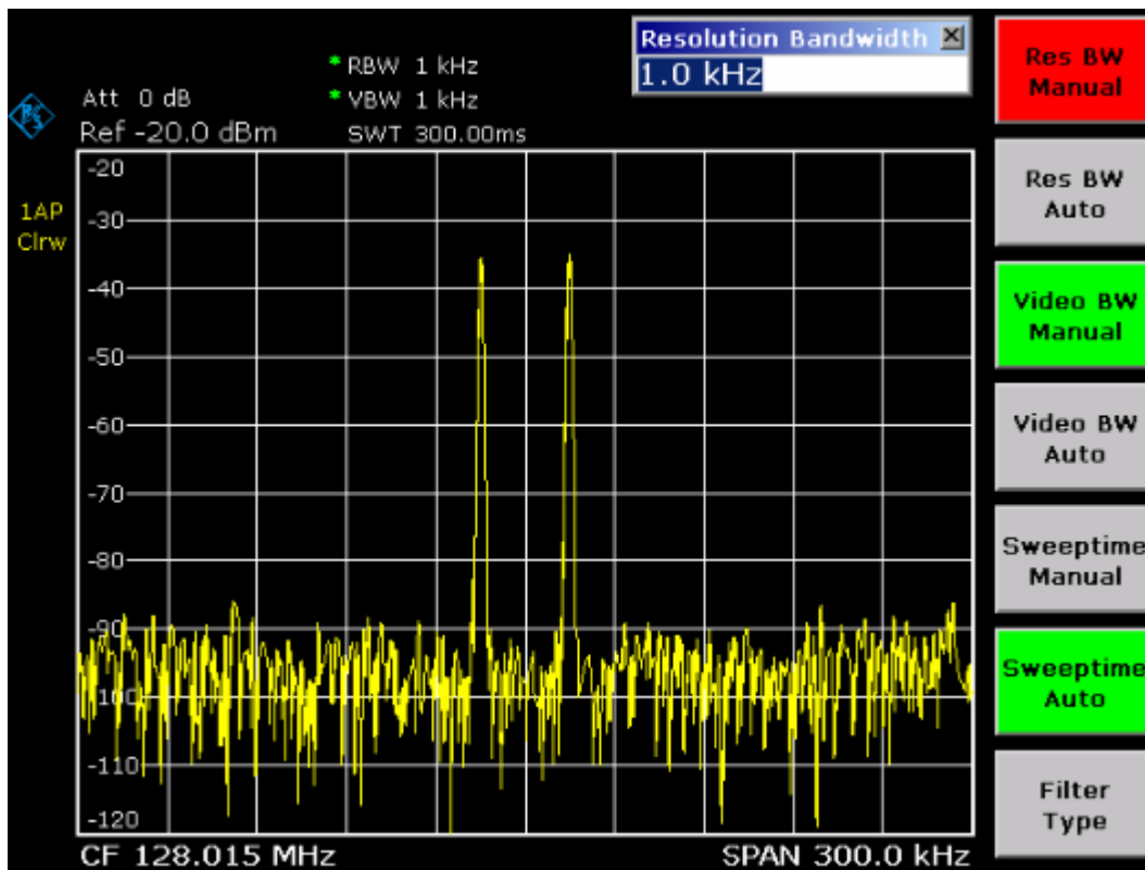
图 5-6 测量两个等电平的射频正弦信号，分辨率带宽（1 kHz）明显小于信号的频率间隔
